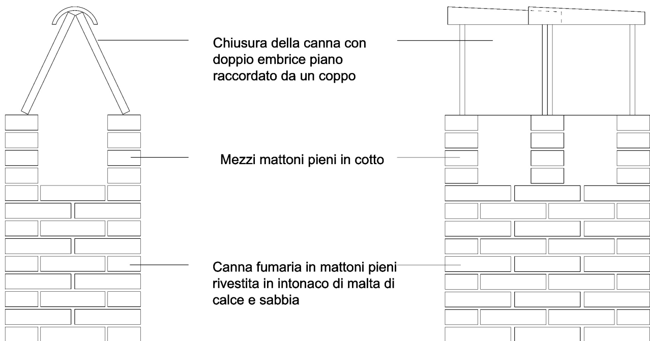
PROSPETTO LATERALE
