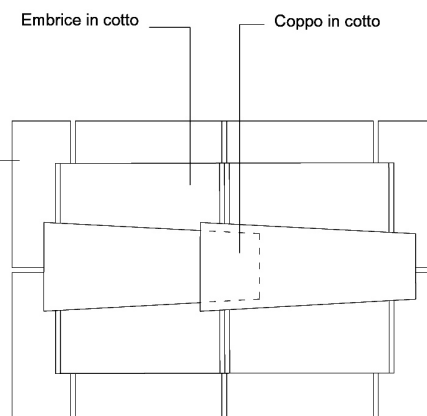
PIANTA LIVELLO COPERTURA
