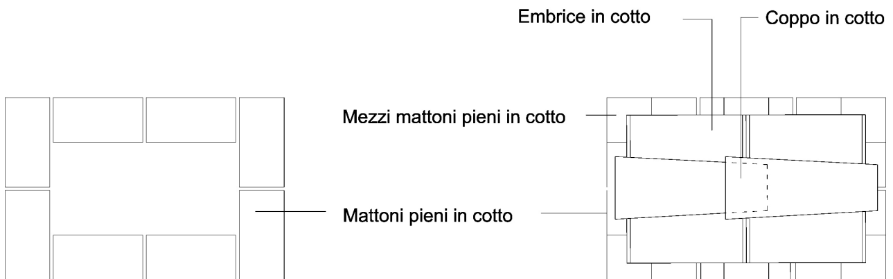
PIANTA LIVELLO MURATURA
